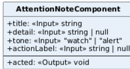
Figura 115: Classe: AttentionNoteComponent
