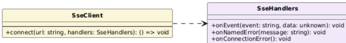
Figura 110: Classe: SseClient
