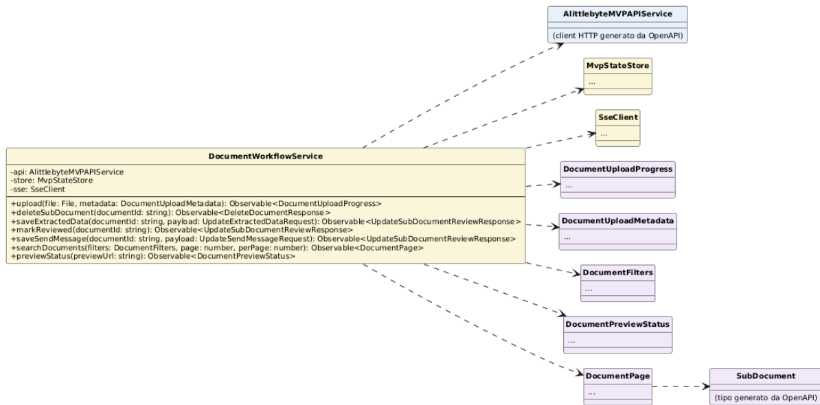
Figura 109: Classe: DocumentWorkflowService
