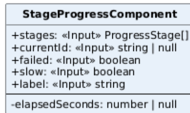
Figura 119: Classe: StageProgressComponent
